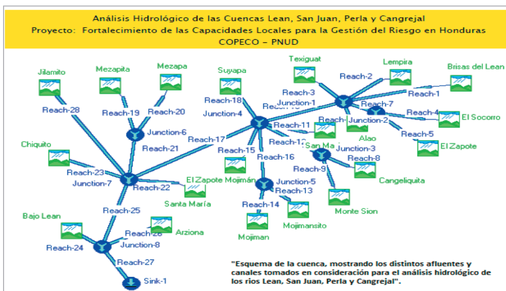
Figura 6 - 4.2.1.1 - Esquema del Modelo HEC-HMS - ríos Lean, San Juan, Perla y Cangrejal
