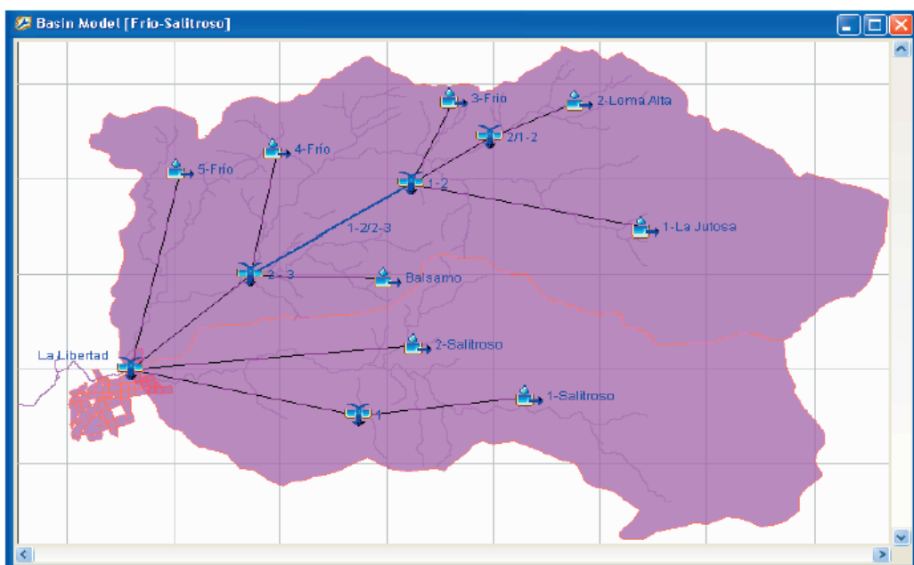
Figura 7 - 4.2.1.2 Esquema del Modelo HEC-HMS Cuencas río Frio y Salitrero
